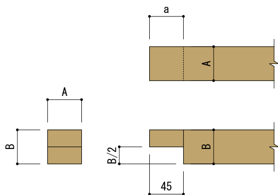
■部材①加工図
