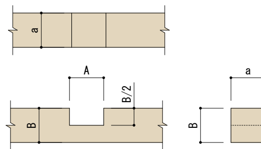
■部材②加工図
