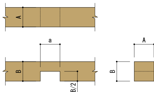
■部材①加工図
