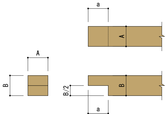
■部材①(男木)加工図
