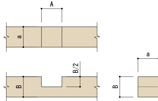
■部材②(女木)加工図
